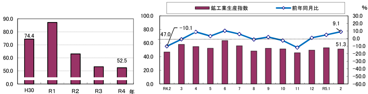
鉱工業生産指数(造船部門)(年別, 月別・前年同月比)
